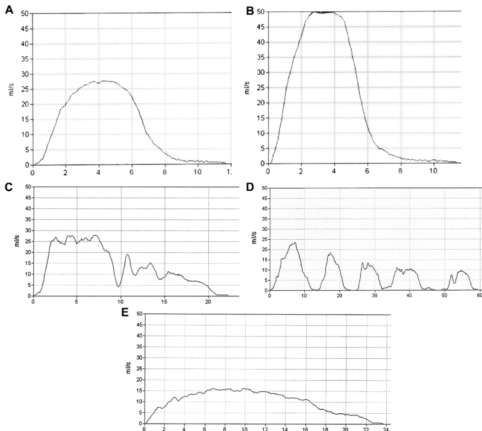
Bild 1. Flödeskurvor (från Austin 2014)
